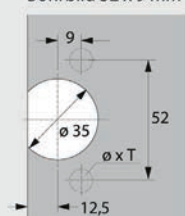
Bohrbild 52 x 9 mm
