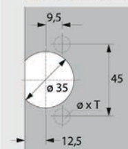
Bohrbild 45 x 9,5 mm
