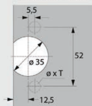
Bohrbild 52 x 5,5 mm
