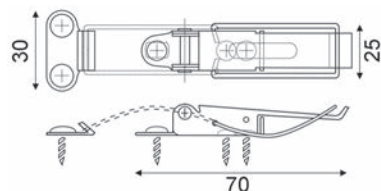
posizione serrato
