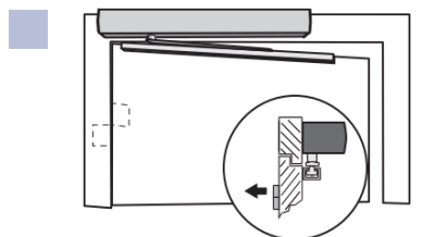
Kopfmontage Bandgegenseite Schiene
