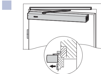
Türmontage Bandseite Schiene
