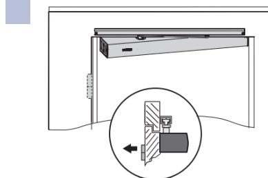
Türmontage Bandgegenseite Schiene
