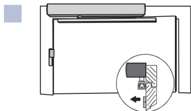
Kopfmontage Bandseite Schiene
