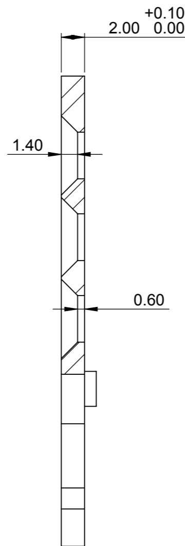
SECTION B-B SCALE 3 : 1
