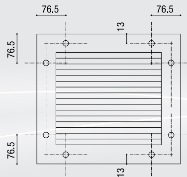
Gitter mit C-Bohrung für nachstehende Größen
