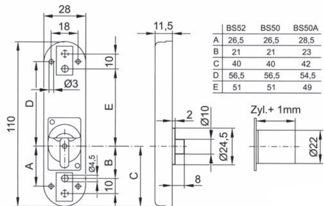
2711 Masszeichnung Dimensions
