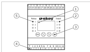
Abb. 5: Übersicht der ekey home SE REG
